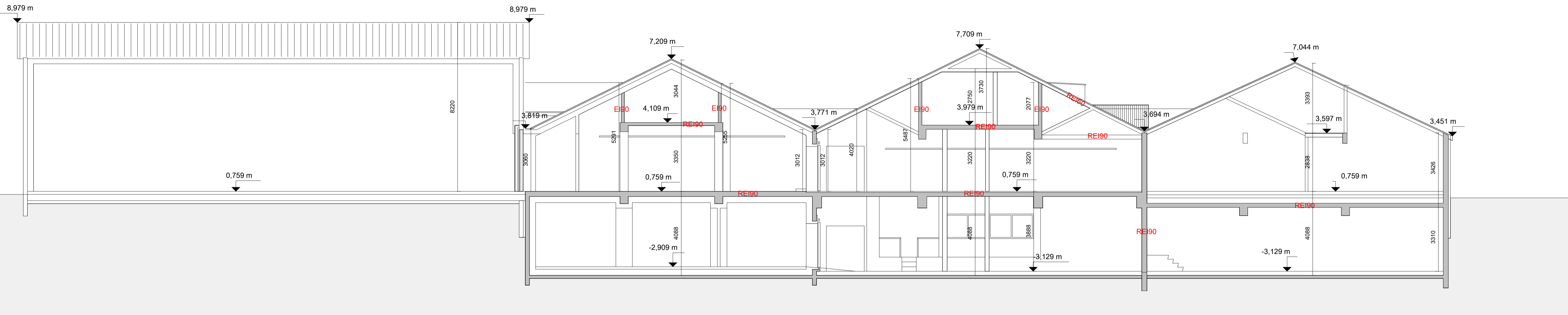
Langsnið 1 mkv: 1 : 100
